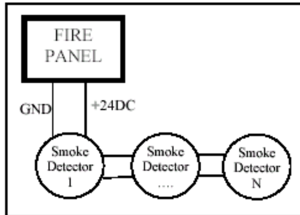
Figura 1 – Conexión típica de un sistema de detectores de Humo.
